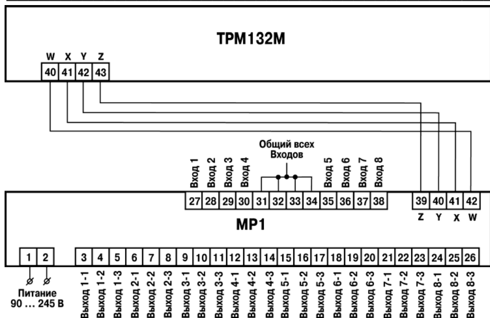
Рисунок Б.1 – Схема подключения ТРМ132М-01 и МР1
